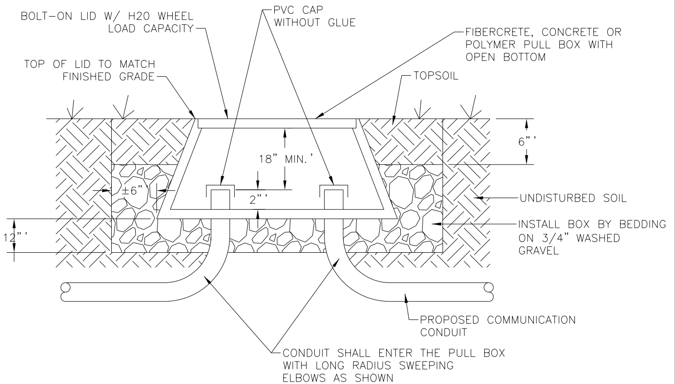
ELEVATION N.T.S.
