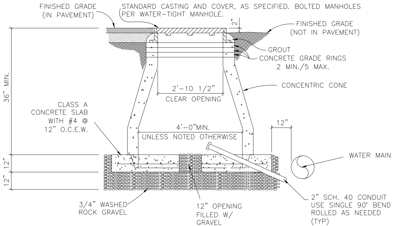
SECTION A-A
