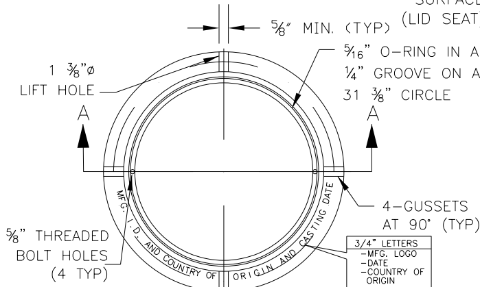
MANHOLE RING
